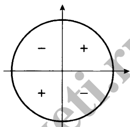
Знаки тангенса
