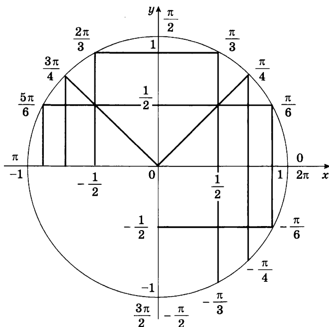
Рис. 3. Тригонометрическая окружность
