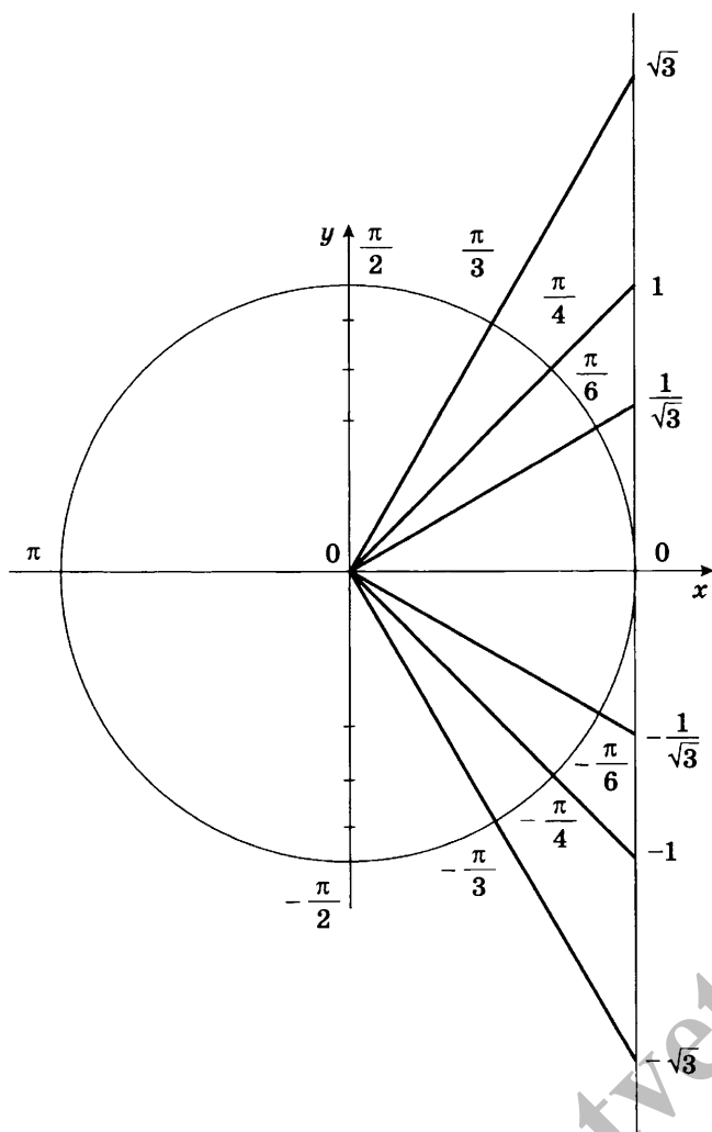
Рис. 6. Линия тангенсов
