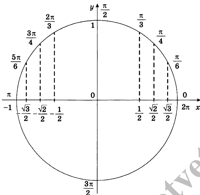
Рис. 5. Линия косинусов
